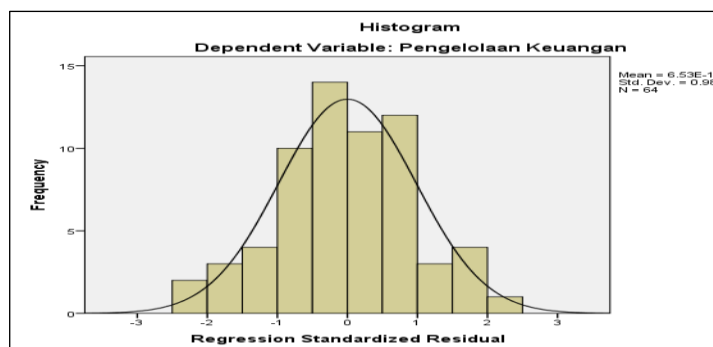
Gambar 1. Histogram Normalitas
